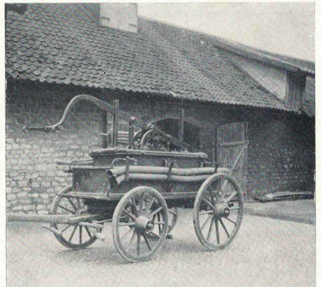
Handdruckspritze aus dem Jahre 1840
